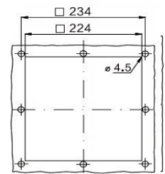
安装开孔图 Cut-out
